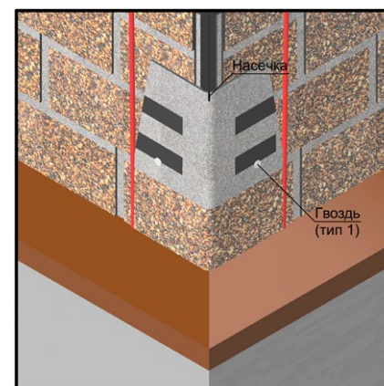
Рис. 20 Фиксация нижнего углового элемента.
